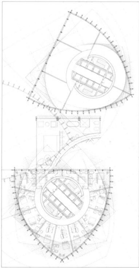
planta tipo (torres) type floor (towers)
