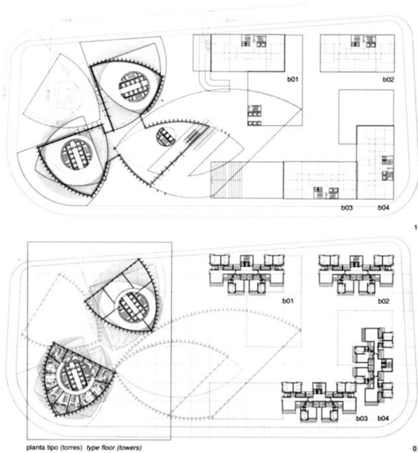
planta tipo (torres) type floor (towers)
